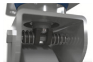
Fjederbelastet retningsbremse
